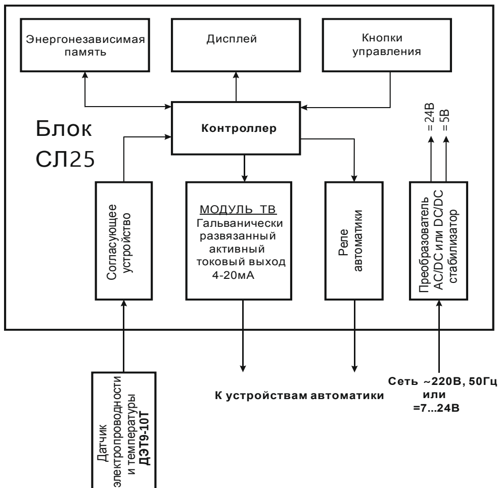
«Блок-схема Блока СЛ25»
