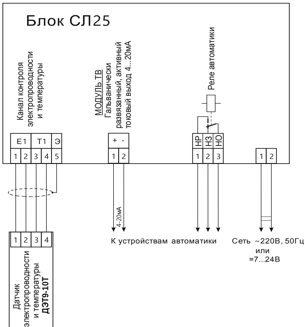
«Схема внешних соединений Блока СЛ25»
