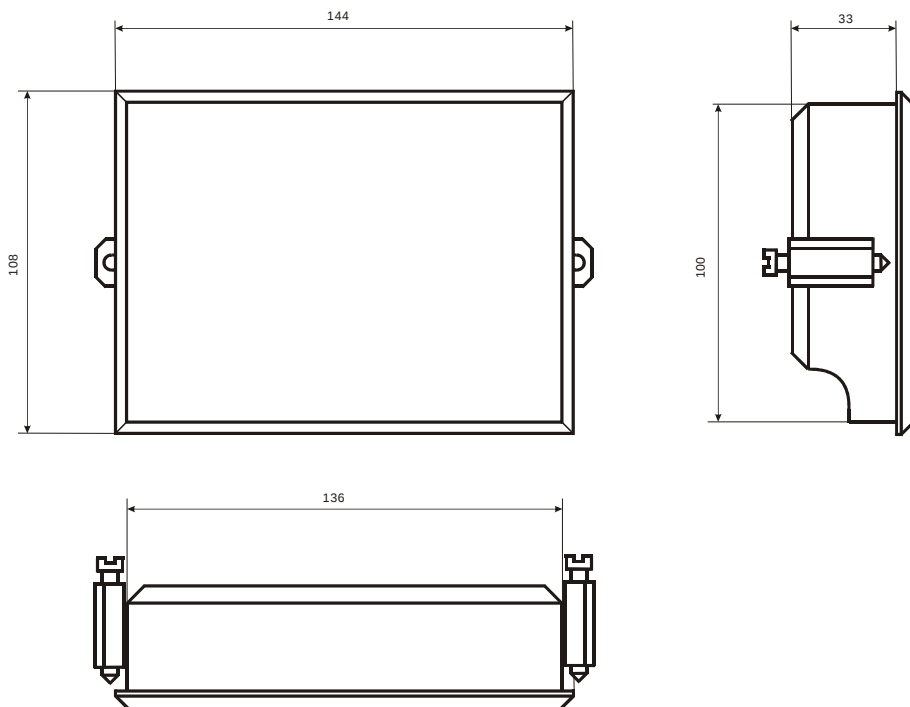
«Габаритные и установочные размеры Блока СЛ25»
